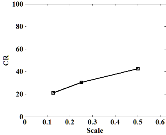
Fig. 6. Correct ratio per Scale.
